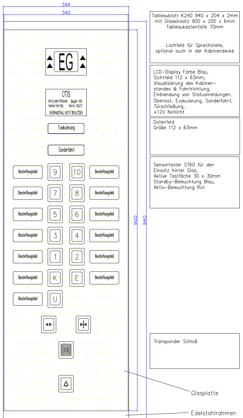
Glastableau mit Außenrahmung V2A K240
